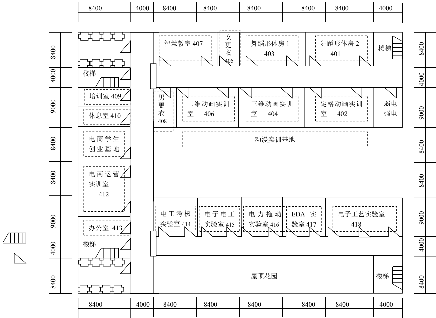
实训楼四层平面图
