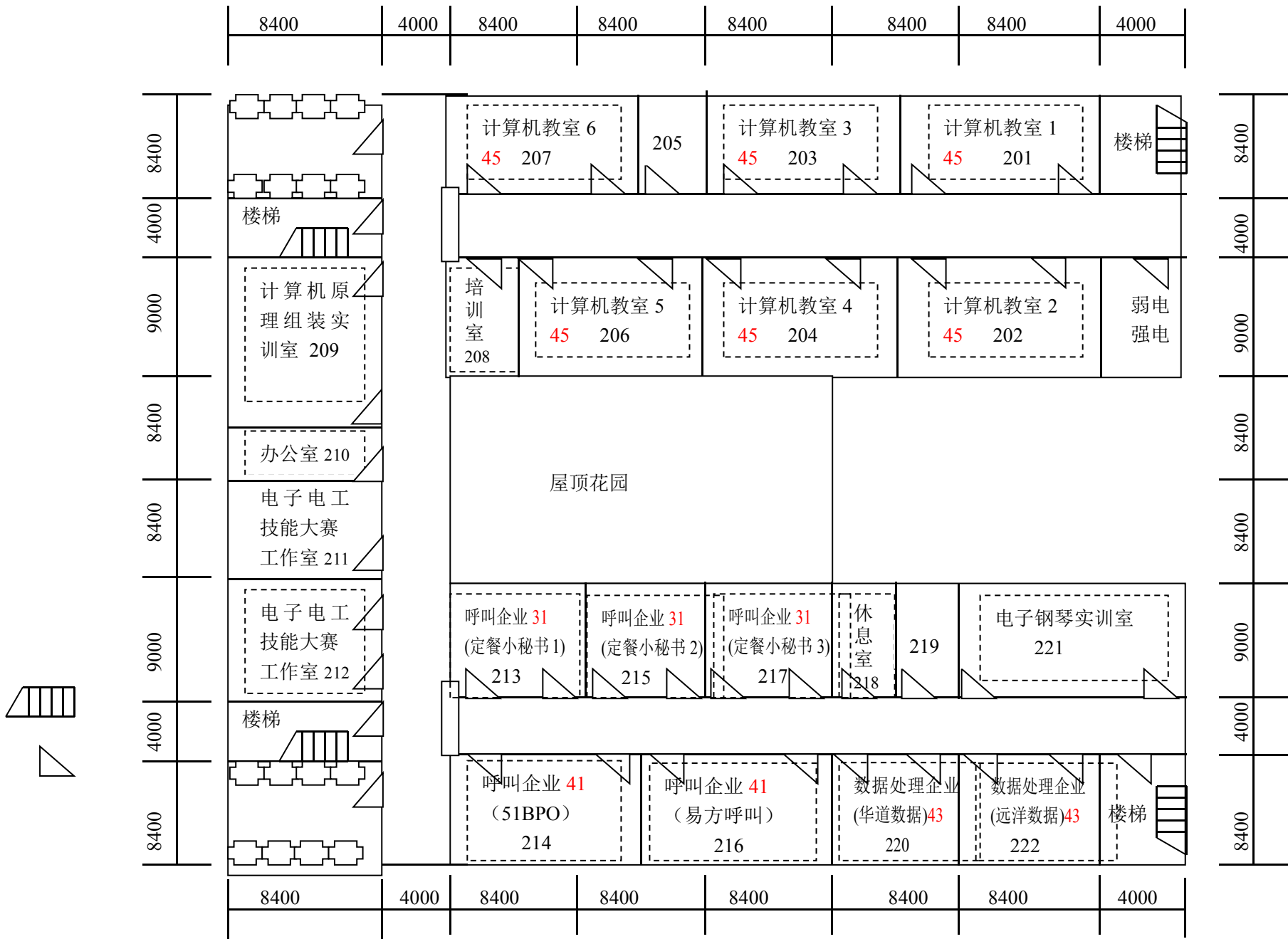
实训楼二层平面图
