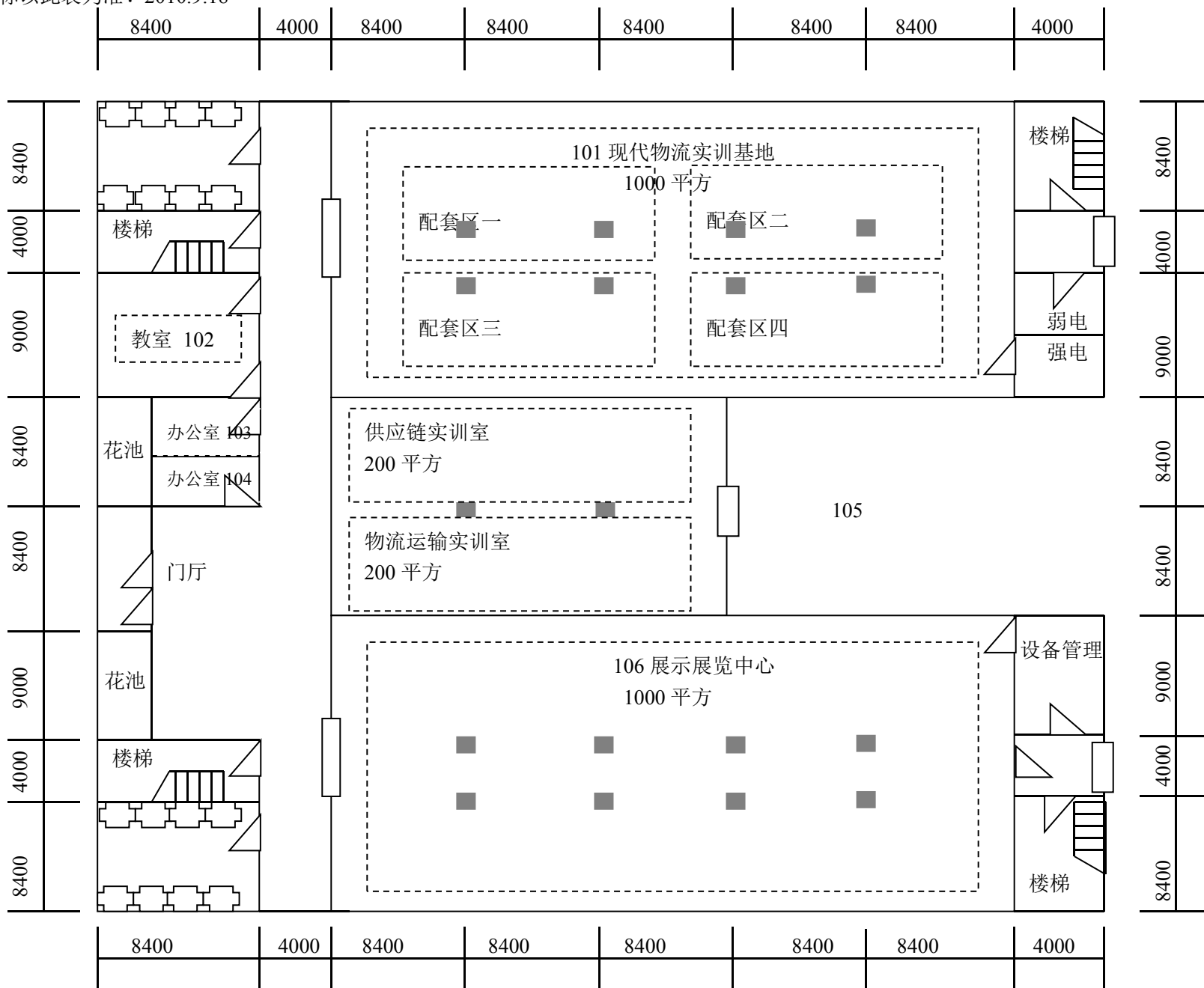
实训楼一层平面图
